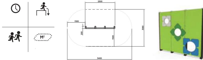
Q13281 Ball Wall 2,4 x 2,2 m
